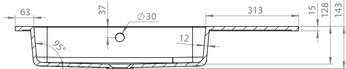
PRZEKRÓJ N-N SKALA 1 : 8
